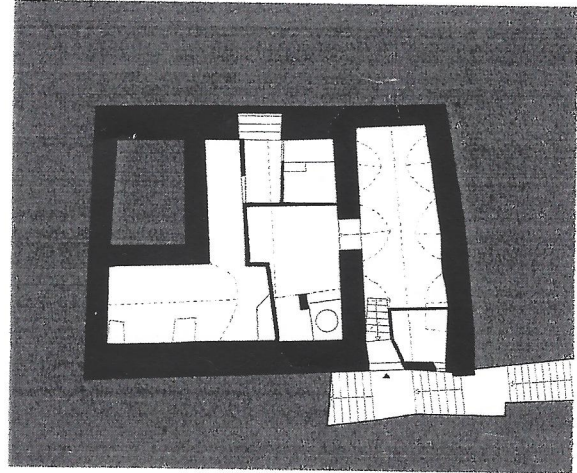
PLAN DU NIVEAU -2
